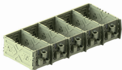
1 ряд - одна общая боковая стенка
